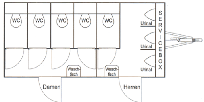
Raumeinteilung WC-Anhänger 5 m
